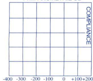
TYMPANOMETRIE OD
